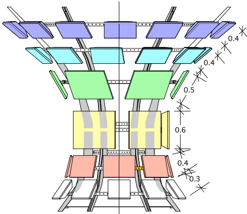
COPAS - ELEVÇÃO - OPÇÃO 2 VISTA COM BACKLIGHT E MONITORES ESC: 1:25
