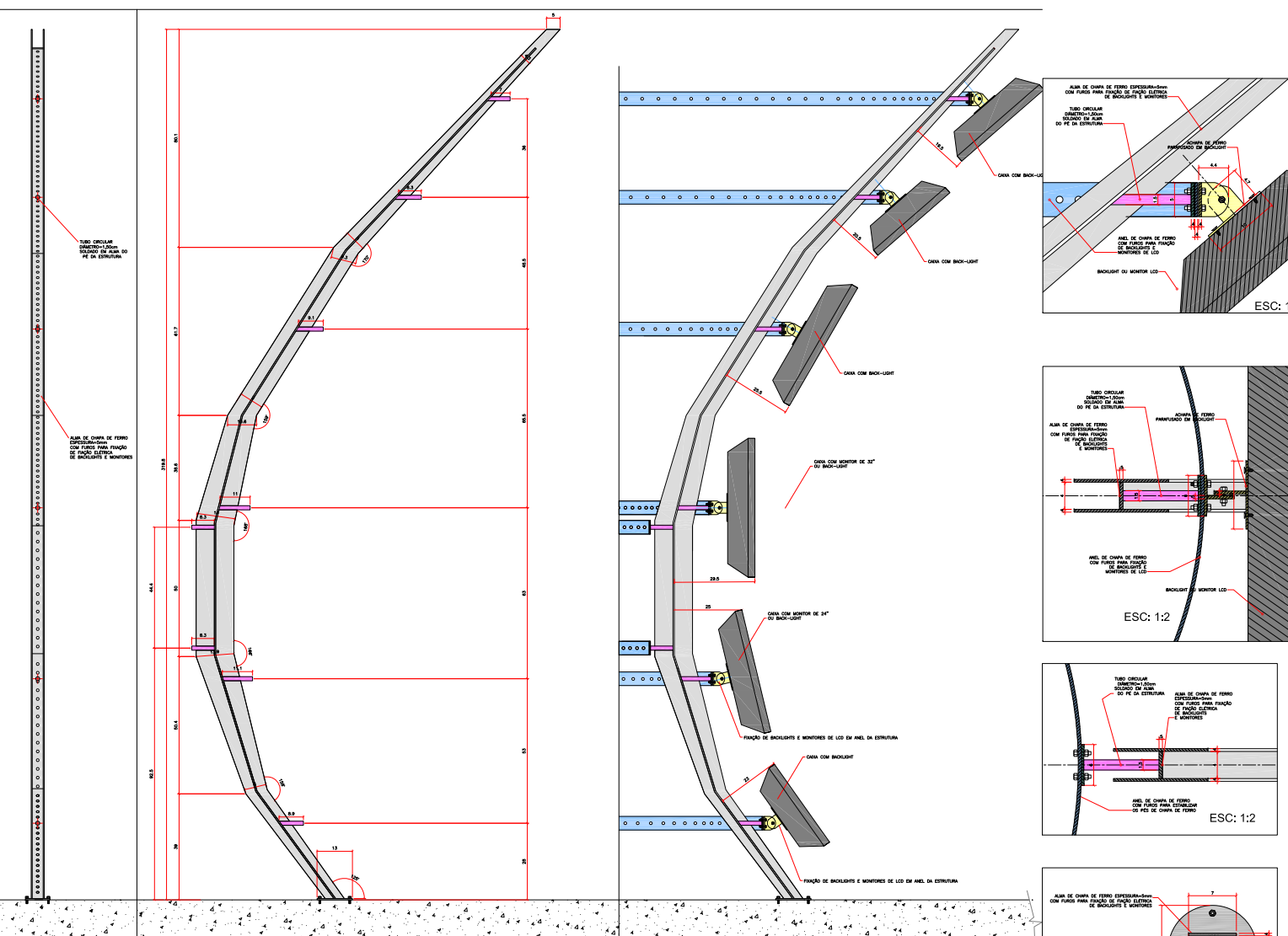
DETALHE COPAS-1 VISTA FRONTAL DE PÉ DA ESTRUTURA ESC:1:5
