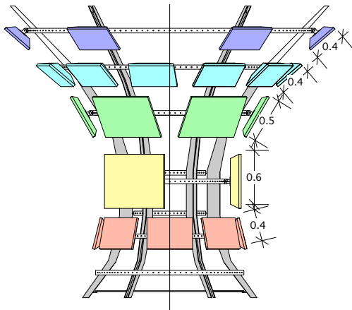
COPAS - ELEVÇÃO - OPÇÃO 1 VISTA COM BACKLIGHT E MONITORES ESC: 1:25
