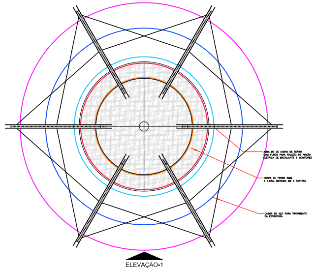
PLANTA DA ESTRUTURA SEM BACKLIGHT E MONITORES ESC: 1:10
